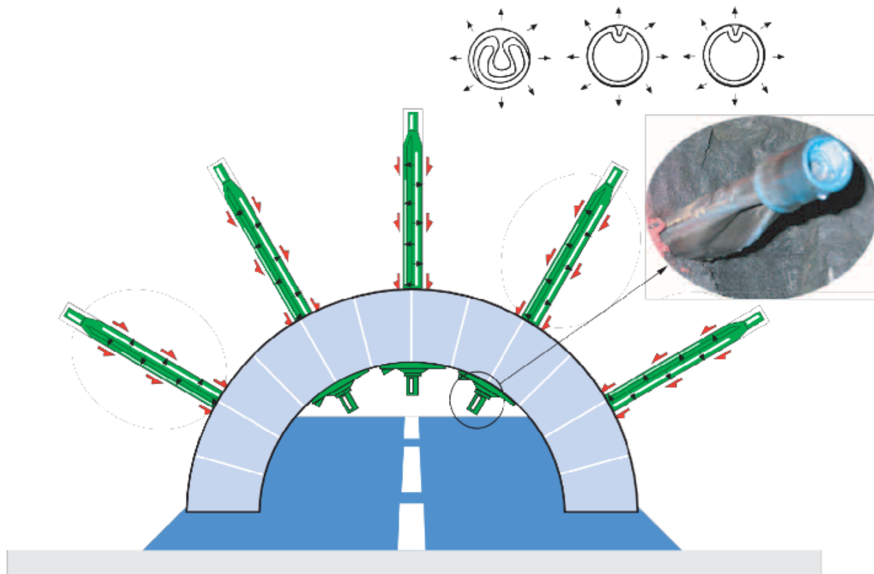
Sostenimiento inmediato radial y por fricción axial L
